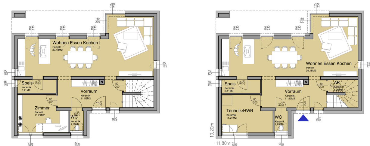
Grundrissvorschlag Erdgeschoss mit und ohne Unterkellerung
