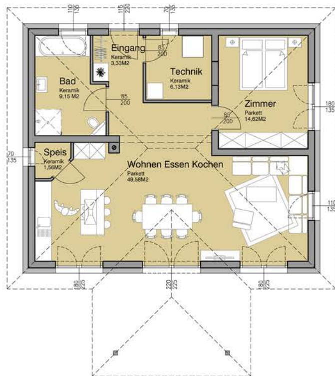
Grundrissvorschlag mit Walmdach
