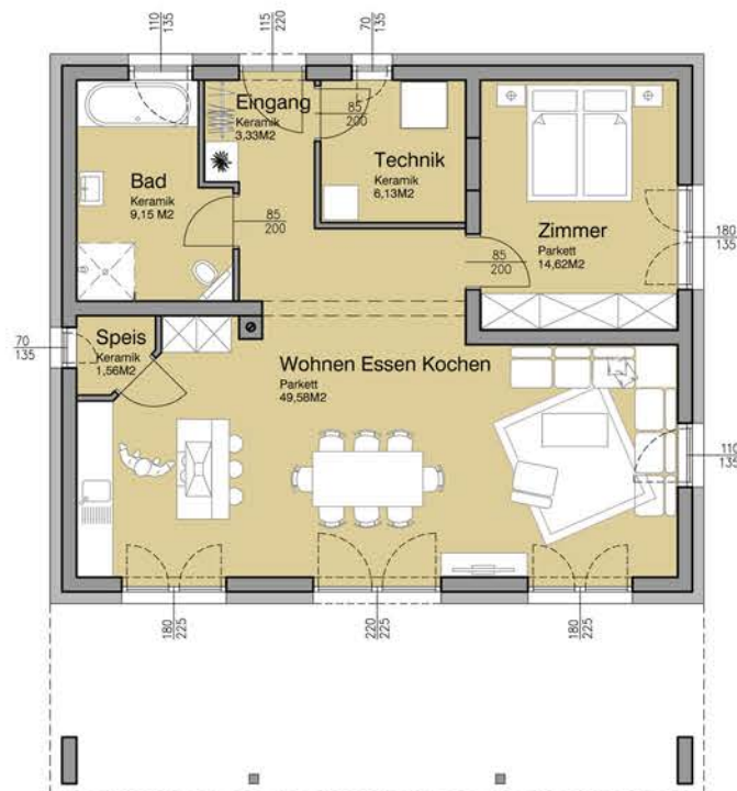
Grundrissvorschlag mit Flachdach
